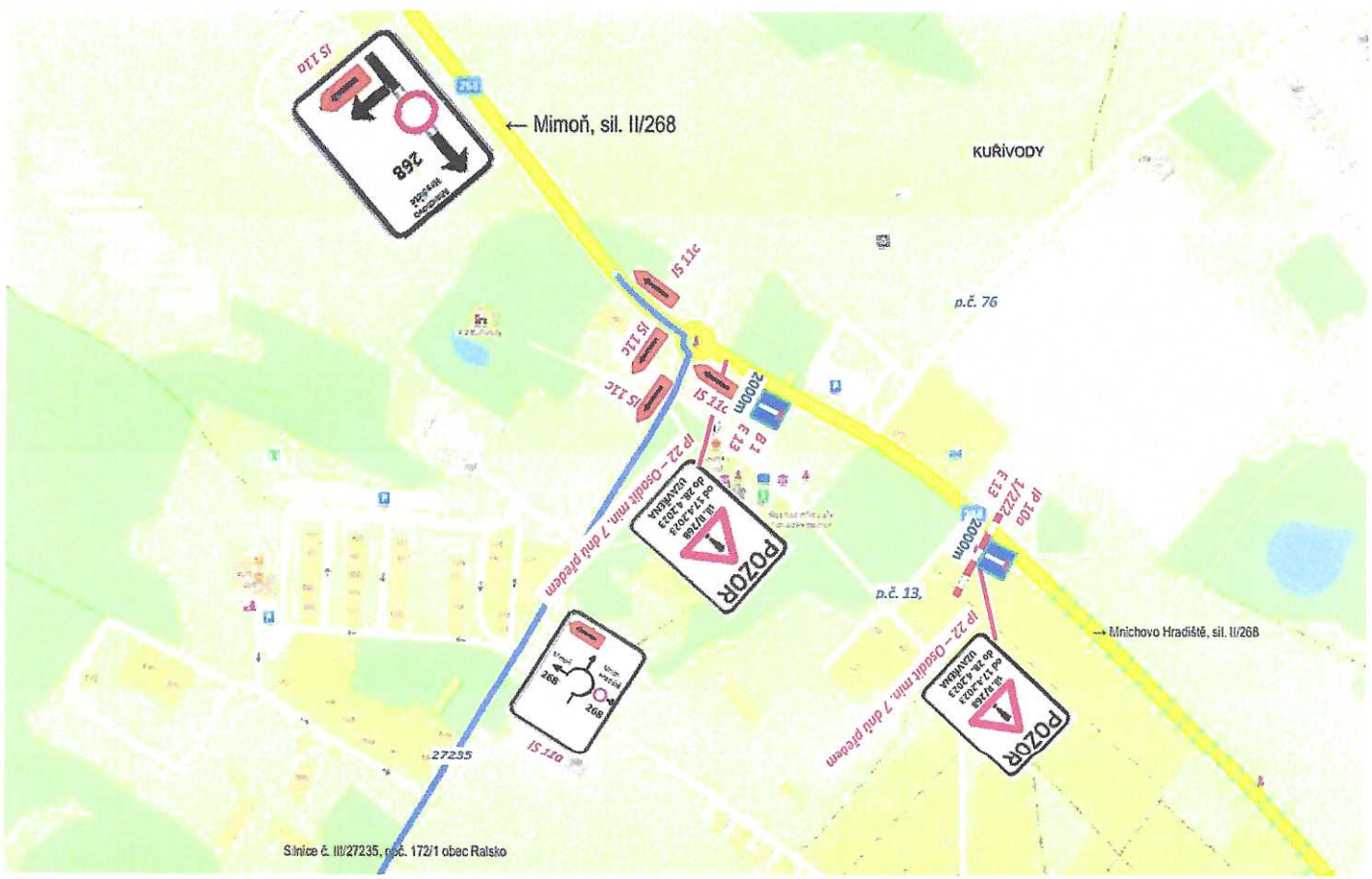
DIO – DETAIL č. 3 – křiž. sil. II/268 a sil. III/27235 - Ralsko
